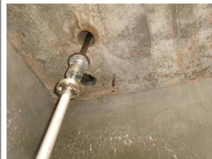
<유출밸브실(2지) 상부슬래브 철근노출>
