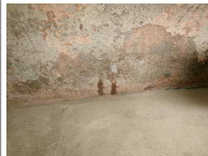
<유출밸브실(1지) 상부슬래브 잠철근노출>
